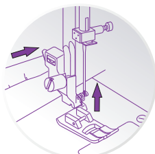
SYSTEM MATIC szybka wymiana stopek
